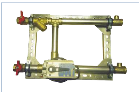
Узел LKG на базе 3-х ходового клапана для холодоснабжения
